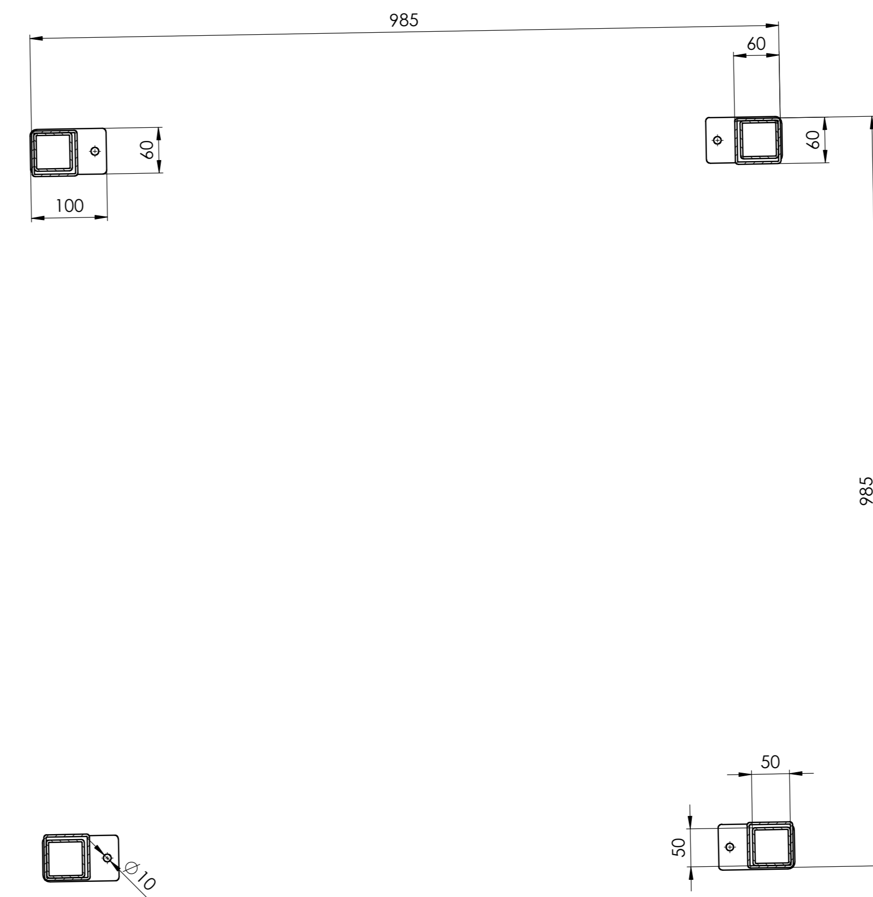
ŘEZ B-B
